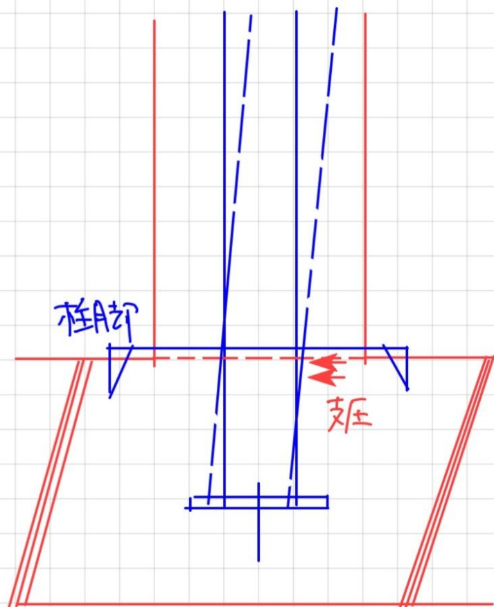
埋め込み型柱脚
